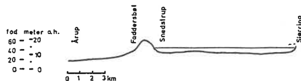
Profil gennem terrænet fra Sjørring sø til Årup mølle langs søens hovedkanal og amtets hovedvandløb nr. 3. Vandspejlet før udtømmelsen er angivet. Konstrueret efter generalstabens målebordsblade 1882-83.
