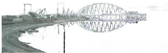
Det første buefag færdigt på Mors-siden.
