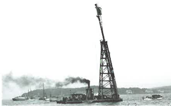
Pælenedramning nærmest Thy-siden.
