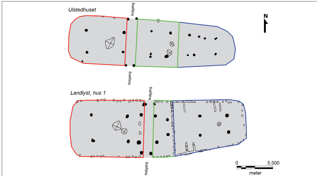
Fig. 4. Sammenligning af husene fra Højgård og Bjerre Enge, efter idé og forlæg af Anne-Louise Haack Olsen
