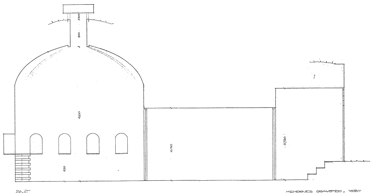
Snittegning af mausoleet i gravhøjen.
