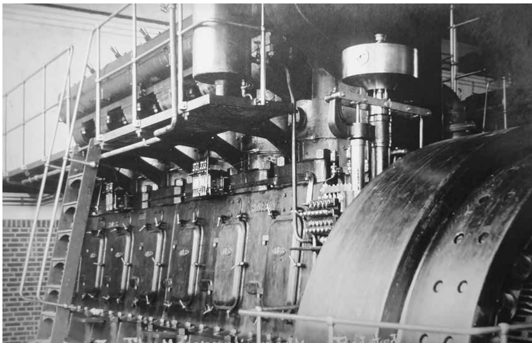
En af selskabets Burmeister & Wain dieselmotorer, som man startede ved hjælp af lufttryk.
