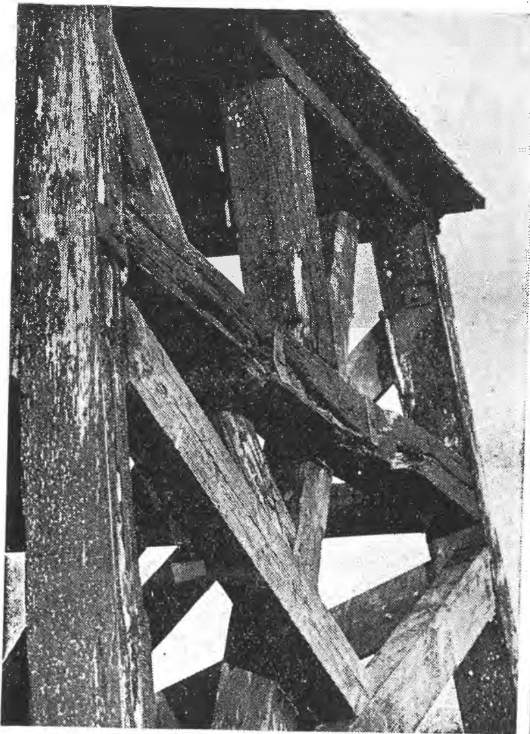
Klokkestabelen, der for længe siden blev fremstillet af skibstømmer, er efterhånden blevet gennemrådden, og skal nu fornyes. Den nye stabel bliver nøjagtig magen til den nuværende, og egeplankerne skal hugges og samles på kirkegården.
