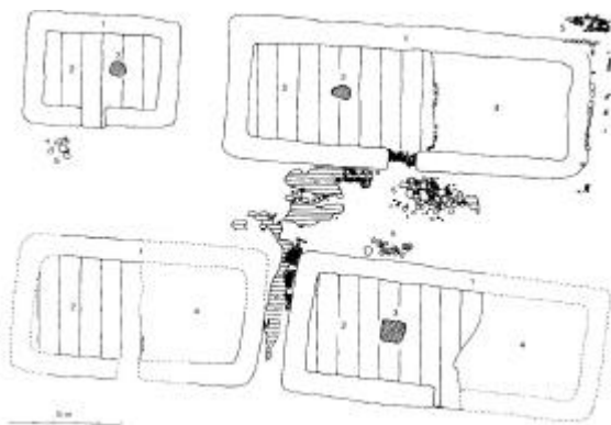
Plan over en del af jernalderbopladsen ved Koldby med 4 huse, der antagelig eksisterede samtidig. 1: Græstørvsvæg. 2: Lergulv. 3: Ildsted. 4: Jordgulv i stald. 5: Stenbrolægning. 6: Lerstampet sti med piksten.
