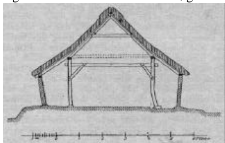
Fig. 1 Tværnsnit af et Hus fra Agger By og Sogn, Refs Herred, Thisted Amt.
