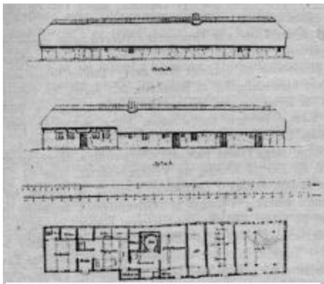
Fig. 2. Hus fra Agger By og Sogn, Refs Herred, Thisted Amt.
