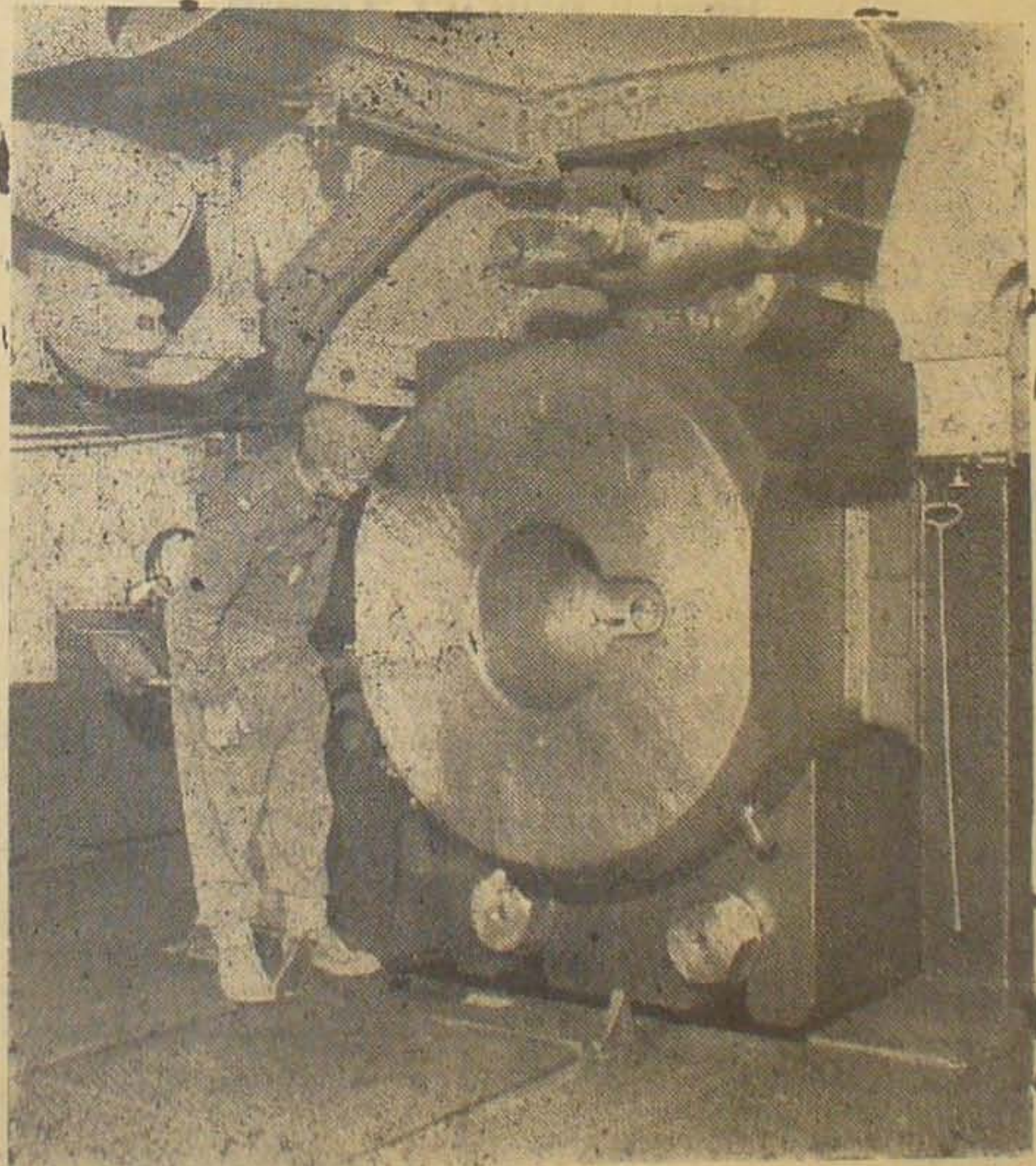
EN AF DE STORE HANSTHOLMKANONER. Vort Billede er hentet inde fra et af Batterierne, hvor man ser Bundstykket af en af de store 38 cm Kanoner.
