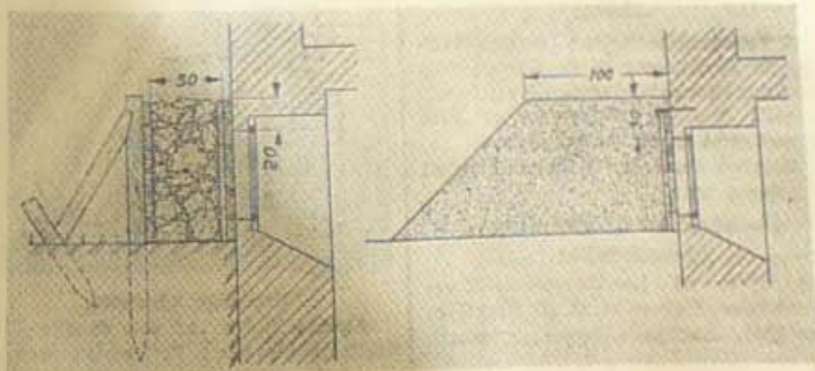
Skitsen ovenfor viser, hvorledes Sikringen bl. a. kan ske. Til venstre ses en Stenpakning afstivet af Bjælker og til højre en Jordvold udenfor Vinduet.
