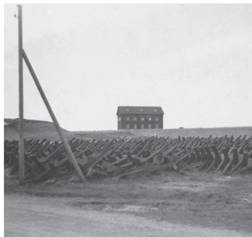
Adskilte panserkryds i den nordlige del af Agger i 1945. Panserkrydsene bestod af tre vinkeljærnsbjælker, hvoraf de to var svejset sammen, mens den tredje var spændt fast til de andre med bolte. De var derfor forholdsvis nemme at transportere og samle på stedet – og siden skille ad igen. Der stod ca. 4000 af dem omkring Agger By. (Lokalhistorisk Arkiv for Thisted Kommune, 4385).
