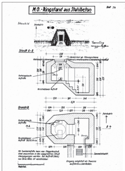
Tysk typetegning af en ringstilling af typen Bauform 58c. Der var 17 små bunkere af denne type omkring Agger By. (Museumscenter Hanstholm)
