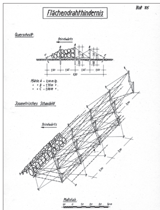
En tysk typetegning af den type pigtrådshegn, som omkransede Agger by. (Museumscenter Hanstholm).
