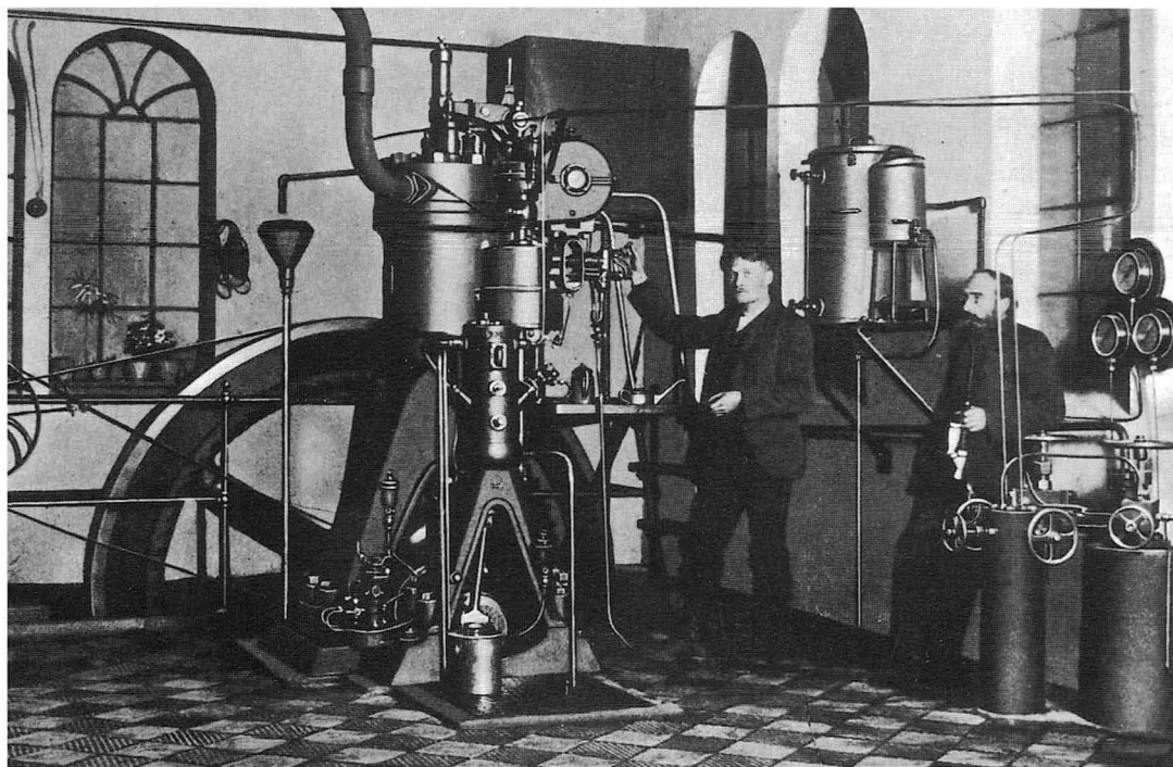
Den 25 HK B&W-motor (den første dieselmotor på et elværk i Danmark) begyndte at producere el til 598 lampesteder den 28. november 1904. Ejeren Kr. Møller (med pibe) ejede elværket til 1913. Personen til venstre er Thorvald Jeppesen, der senere blev den første bestyrer af elværket (1913-1931).
