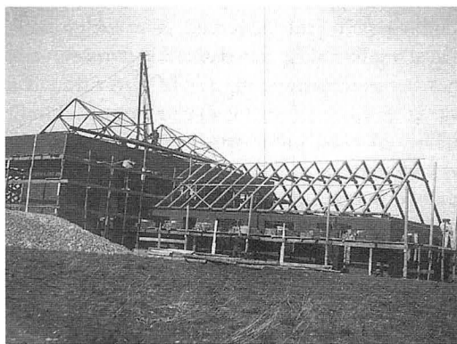
Min første store opgave som værkfører var at lave stålspærrene til maskinhallen ved Hurups nye elværk. Foto 1947.
