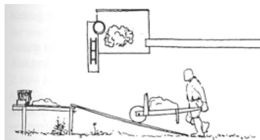
Strygebord, set ovenfra og fra siden. Fra æltegraven kørtes leret, der nu havde konsistens som tyk bankerot (= mørtel), til strygebordet, hvor »strygeren« med hurtige hænder kastede to håndfulde ler i forme og strøg det overskydende ler af, inden den våde sten blev lagt til tørring på jorden et par dage. Herfra kørtes stenene til tørreladerne for til sidst at blive stablet i ovnen til brænding
