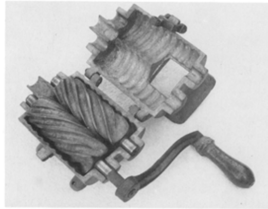
Kødhakkemaskine. Fabrikationsnr. 126, men fra hvilken fabrik?
