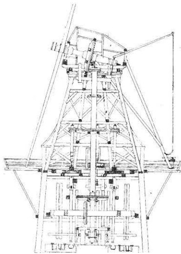
Jes Thiesens konstruktionstegning til vindmølle.
