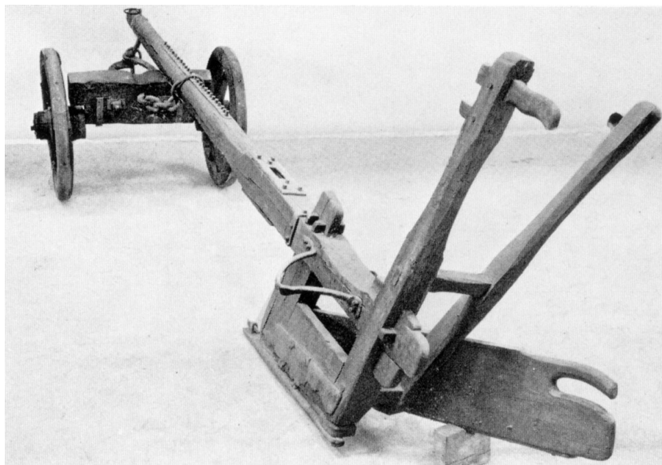
Hjulplow fra Nors.
